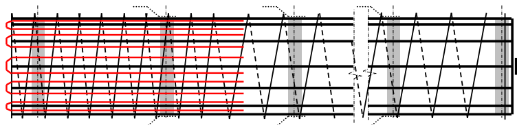
Standard Pfahlkorb mit Kopfverbügelung
