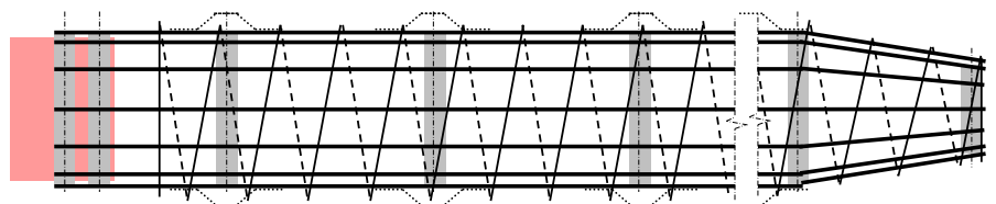
D0_Pfahl mit Rüttelklinge und Korbverjüngung
