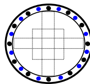
A1_Pfahlkorb mit aussenliegenden Zulagen
