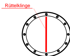
D0_Pfahl mit Rüttelklinge und Korbverjüngung
