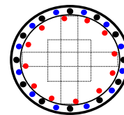
A2_Pfahlkorb mit aussen- und innenliegenden Zulagen
