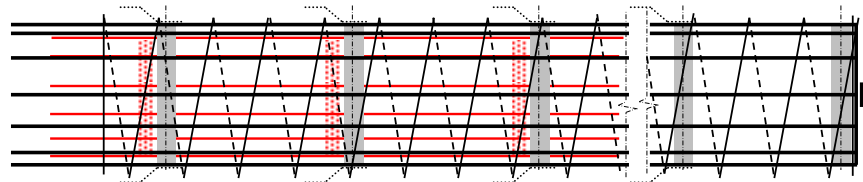
Standard Pfahlkorb mit Kopfverbügelung
