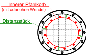
B0_Pfahl in Pfahl
