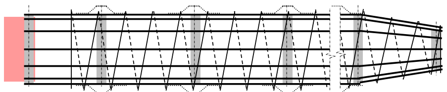
D0_Pfahl mit Rüttelklinge und Korbverjüngung
