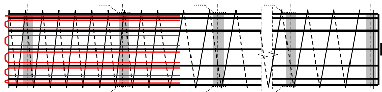
Standard Pfahlkorb mit Kopfverbügelung
