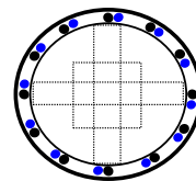
A2_Pfahlkorb mit aussenliegenden Zulagen als Doppelstab
