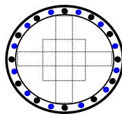
A1_Pfahlkorb mit aussenliegenden Zulagen in Stablücke
