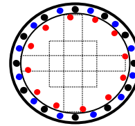
A2_Pfahlkorb mit aussen- und innenliegenden Zulagen
