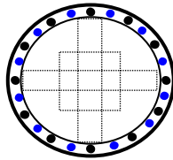
A1_Pfahlkorb mit aussenliegenden Zulagen
