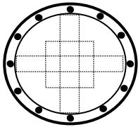
A0_Pfahlkorb Standard
