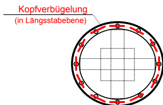
C0_Köcher-Pfahlkorb Standard Pfahlkorb mit Kopfverbügelung
