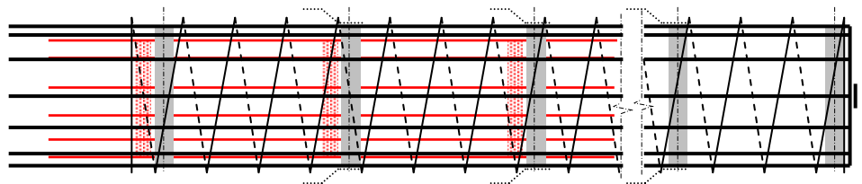
B0_Pfahl in Pfahl Standard Pfahlkorb mit innenliegendem Pfahlkorb
