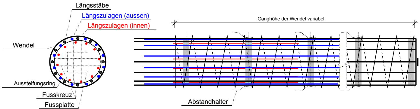
A0_Pfahlkorb Standard
