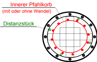
B0_Pfahl in Pfahl Standard Pfahlkorb mit innenliegendem Pfahlkorb
